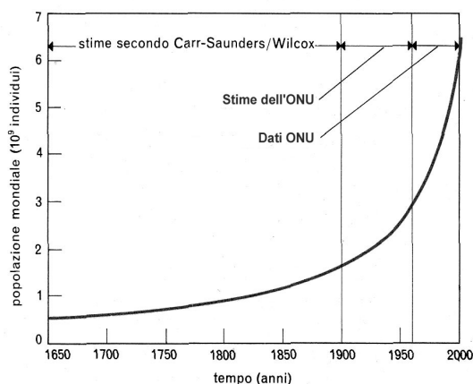
Figura 2. La curva della popolazione mondiale si sovrappone quasi esattamente (per lo stesso periodo esaminato) a quella della produzione industriale USA. Per avere un accenno di flesso occorreranno un paio di generazioni.
