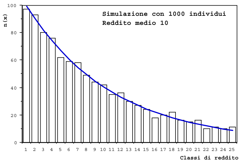
Figura 12. Distribuzione del reddito ottenuta dopo 100.000 interazioni per un sistema composto da 1.000 individui e con ricchezza media 10. Si osservi l'andamento fluttuante intorno alla curva esponenziale teorica che interpola il risultato della simulazione.
