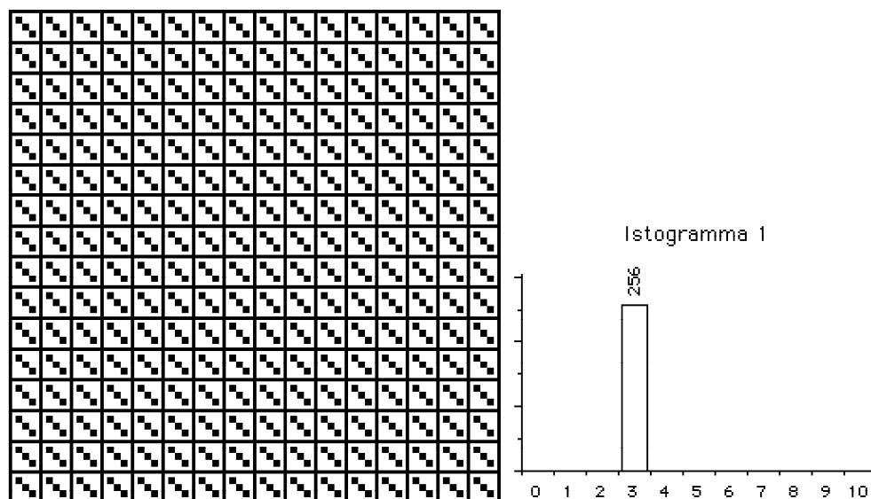
Figura 8. Situazione di partenza, distribuzione uniforme della ricchezza.
