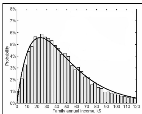
Figure 15 e 16. Reddito individuale e delle famiglie in USA nel 1996 (in verticale le percentuali della distribuzione). Istogrammi ricavati dai dati empirici e curve teoriche sovrapposte. Nel primo caso la realtà mostra un'esponenziale approssimata; nel secondo una classica curva di Pareto quasi perfettamente sovrapposta. Le ragioni di questa differenza qualitativa sono controverse: dal punto di vista puramente fisico essa indicherebbe un comportamento casuale (entropico) dei singoli agenti e un comportamento governato da rovesciamento della prassi nelle loro famiglie (cfr. Dragulescu-Yakovenko).
