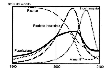
Figura 7. Andamento dei fattori della produzione con la proiezione dei dati 1992 ma con l'ipotesi che dal 1995 una politica demografica permetta di limitare le nascite a due figli per coppia (stabilità della popolazione mondiale).
