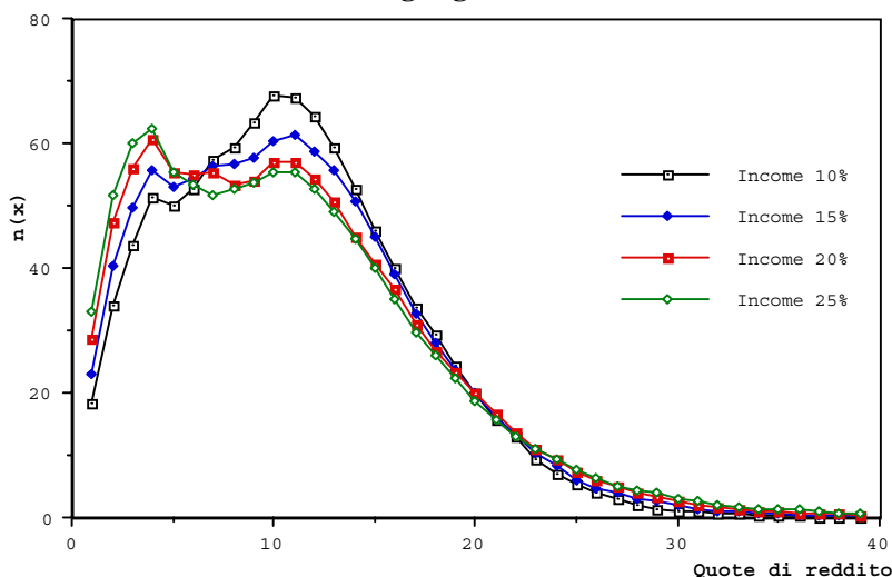
Figura 21. Distribuzione del reddito in presenza di prelievi fiscali dal 10 al 25%. Le varie curve dipendono assai poco da tali coefficienti.
