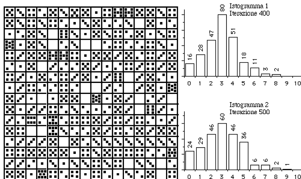
Figura 9. Situazione dopo 500 interazioni (istogramma 2): l'andamento è già asimmetrico. Notare che all'iterazione 400 la distribuzione ha mostrato temporaneamente una curva quasi gaussiana (a campana).
