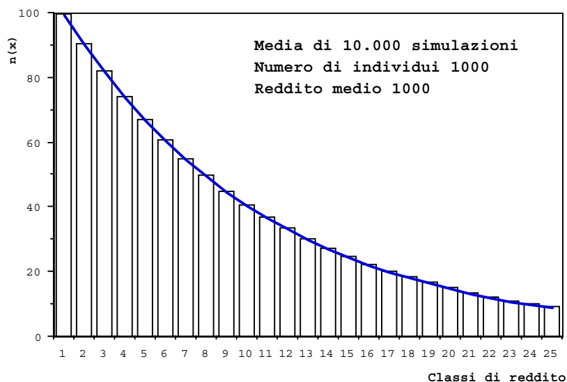
Figura 13. Media di 10.000 istogrammi registrati in simulazioni diverse dopo che si è raggiunta la situazione di equilibrio data in figura 5. Il risultato statistico approssima perfettamente la curva esponenziale teorica.
