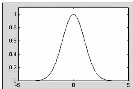
Figura 4. Curva di Gauss "a campana".
