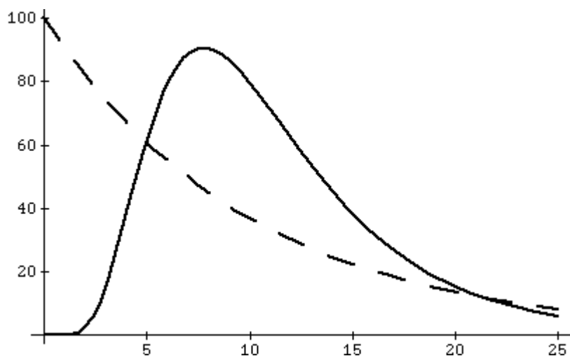
Figura 14. Rappresentazione grafica di una distribuzione di reddito teorica caratterizzata da una curva basata non sul reddito ma sul suo logaritmo. Il numero dei percettori è 1000 e il valore medio del reddito percepito 10.
