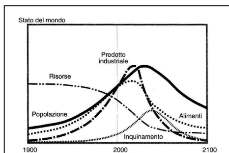
Figura 6. Andamento dei fattori della produzione con la semplice proiezione dei dati 1992.
