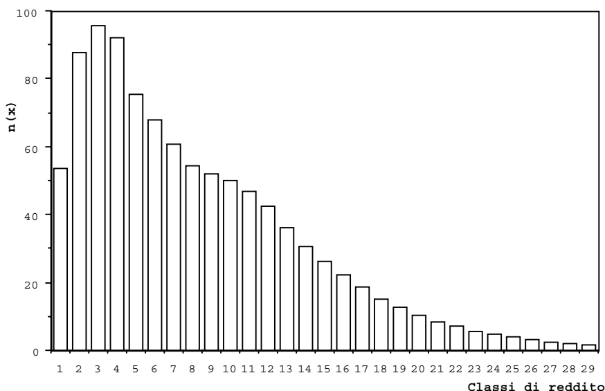
Figura 23. Istogramma della distribuzione del reddito nell'ipotesi che l'economia sia in recessione con una contrazione del 3%.
