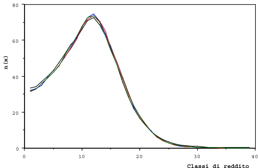
Figura 20. Curve di distribuzione del reddito ottenute con una imposizione del 10% ed assumendo una evasione fiscale crescente per redditi pari a 1, 2, 3, 4 volte il reddito medio. La distribuzione non è praticamente sensibile a questo parametro tipico della demagogia "riformista" e le diverse curve quasi si sovrappongono.
