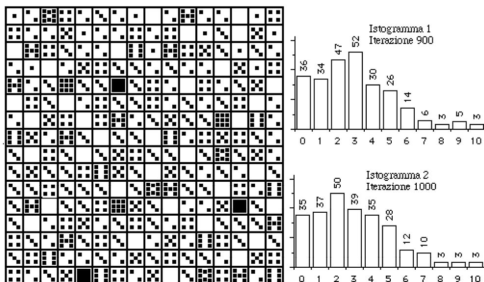
Figura 10. Dopo 900 interazioni (istogramma 1) e 1000 (istogramma 2 e quadrato grande) la curva diventa decisamente asimmetrica. La rappresentazione "sociale" implicita nel quadrato grande mostra già 35 caselle vuote (con ricchezza nulla) e 3 caselle piene (con reddito accumulato = ricchezza maggiore di 9).
