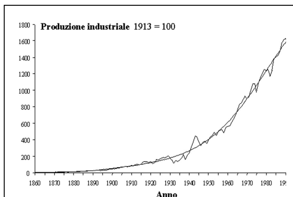
Figura 1. Indice della produzione industriale USA 1860-1990. La curva regolarizzata presenta un andamento esponenziale nel primo tratto e un flesso negli anni '70, con una tipica forma a "S". Dati recenti mostrerebbero un più visibile andamento asintotico nell'ultima parte. È interessantissimo notare come in singoli frammenti di curva si presenti una forma "frattale", vale a dire che ogni singolo periodo contiene una forma invariante rispetto all'intero corso storico esaminato. Proprio da osservazioni del genere Benoît Mandelbrot trasse spunto per avviare i suoi studi matematici sui frattali (fonte: Dinamica dei processi storici – Teoria dell'accumulazione , Quaderni di n+1 1992).
