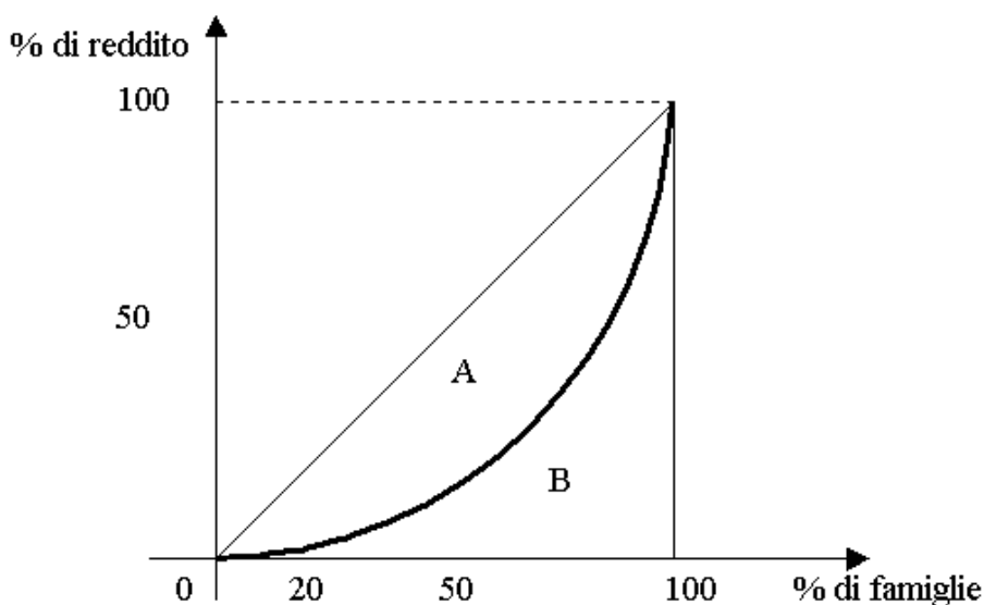
Figura 18. Curva di Lorentz.
