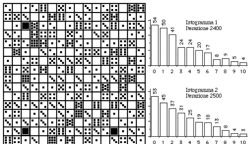
Figura 11. Dopo 2400 interazioni (istogramma 1) la distribuzione è già esponenziale, con qualche fluttuazione. Dopo 2500 (istogramma 2 e quadrato grande) l'andamento esponenziale è netto con ammassamento a reddito zero e "coda" verso reddito dieci.
