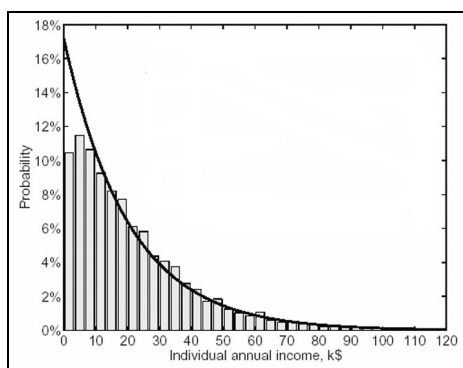
Figure 15 e 16. Reddito individuale e delle famiglie in USA nel 1996 (in verticale le percentuali della distribuzione). Istogrammi ricavati dai dati empirici e curve teoriche sovrapposte. Nel primo caso la realtà mostra un'esponenziale approssimata; nel secondo una classica curva di Pareto quasi perfettamente sovrapposta. Le ragioni di questa differenza qualitativa sono controverse: dal punto di vista puramente fisico essa indicherebbe un comportamento casuale (entropico) dei singoli agenti e un comportamento governato da rovesciamento della prassi nelle loro famiglie (cfr. Dragulescu-Yakovenko).
