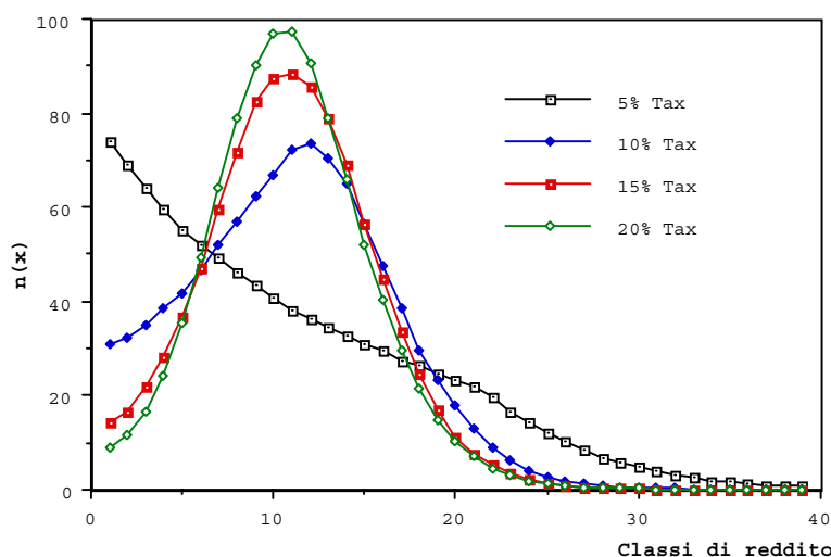
Figura 19. Curve di distribuzione con una pressione fiscale del 5, 10, 15, 20 % e con una redistribuzione statisticamente uniforme del prelievo fiscale.
