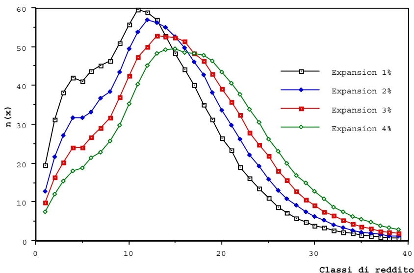
Figura 22. Distribuzione del reddito in una economia con un tasso di espansione dell'1, 2, 3, 4% e con tassazione pari al 10%. Le curve si modificano, ma non in modo sostanziale.
